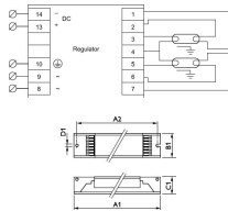
Technische Daten Philips HF-R 258 TL-D EII 220-240V für 2x58W
