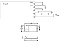
Technische Daten Philips Kugelast HID-AV C 35-70 / I CDM 220-240V 50/60Hz
